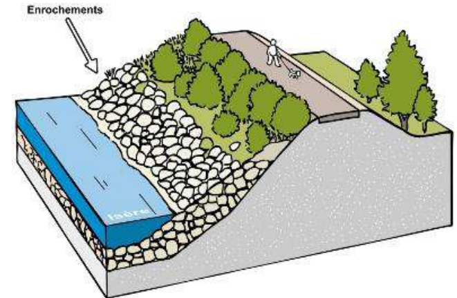
Illustration d'une digue – source AD Isère Drac Romanche
