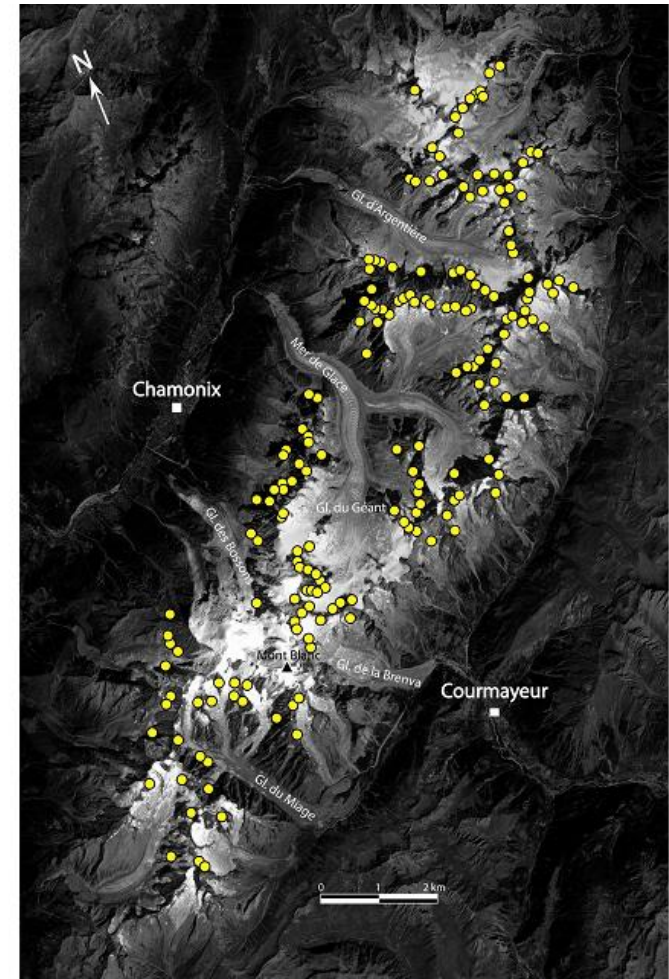
Fig. 8.14 – Position des 182 écoulements de 2003 sur un secteur de l'image satellite SPOT-5 panchromatique 051/257 du 23 août 2003 (10 h 50 TU). Position of the 182 rockfalls of 2003 on a sector of the panchromatic SPOT-5 satellite image 051/257 of the 23 August 2003 (10:50 GMT).
