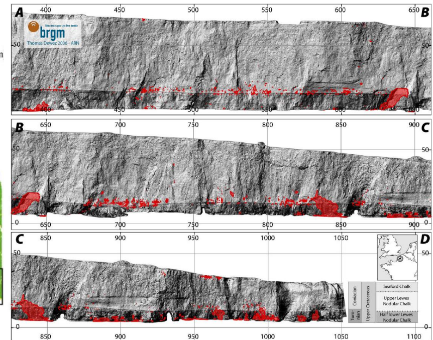
Falaise de còtière de Mesnil Val, Haute-Normandie (Dewez et al, 2009).
