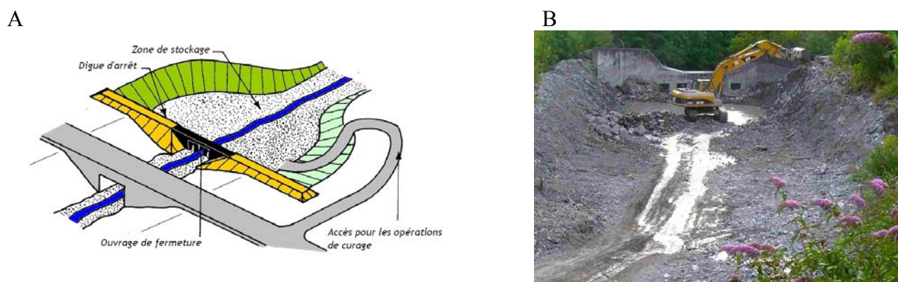
Figure 2. (A) Schéma de principe d'une plage de dépôt (Van Dine, 1996) ; (B) opération de curage mécanique d'une plage de dépôt sur un torrent isérois (photo : Pascal Diot)
