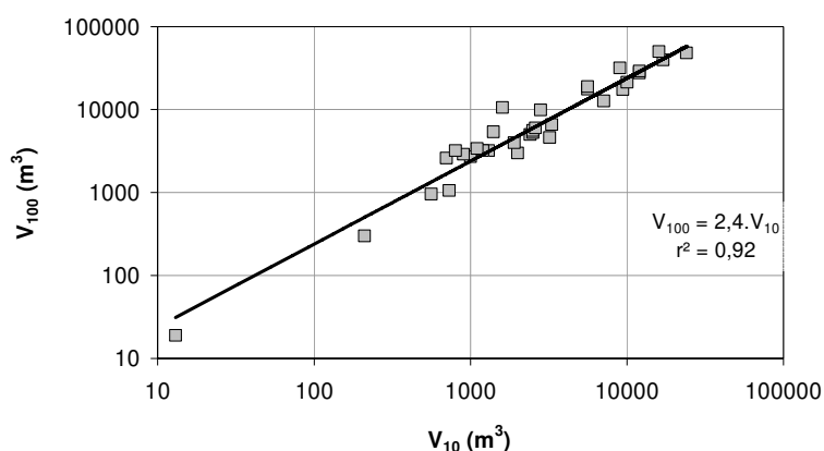
Figure 9. Graphe de corrélation entre le volume solide décennal et centennal
