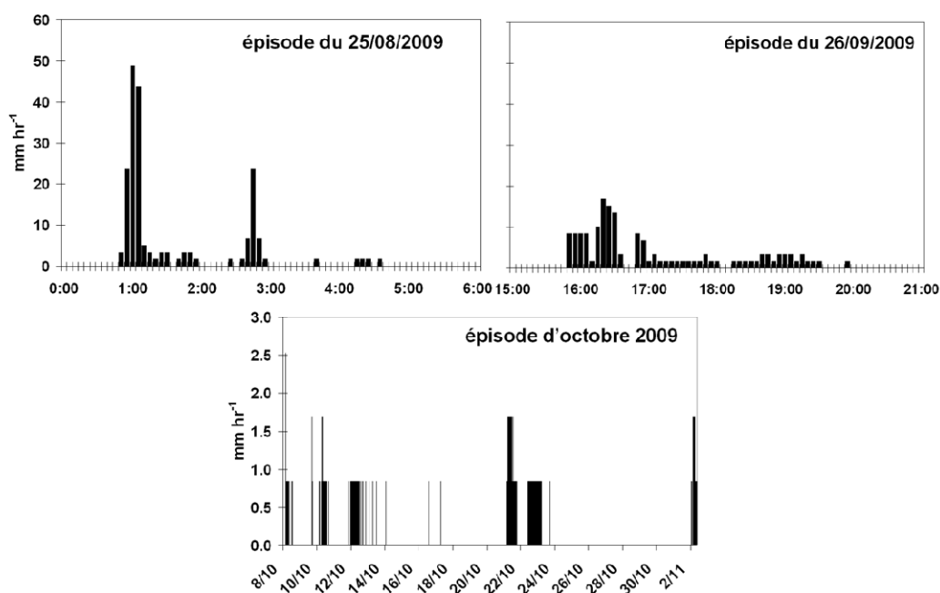
Figure 24. Hyetogrammes des épisodes pluvieux d'août, septembre et octobre 2009 mesurés dans le haut bassin du Manival (intensités mesurées selon un pas de temps de 5 mn)
