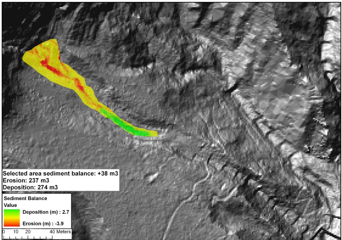
Figure 29. Distribution spatiale de l'érosion et du dépôt obtenue par LiDAR terrestre sur la ravine M1 après l'événement du 25/08/2009 ; on voit que les déstabilisations linéaires proximales se sont déposées à proximité des zones de départ et que les matériaux n'ont pas transité jusqu'au chenal principal
