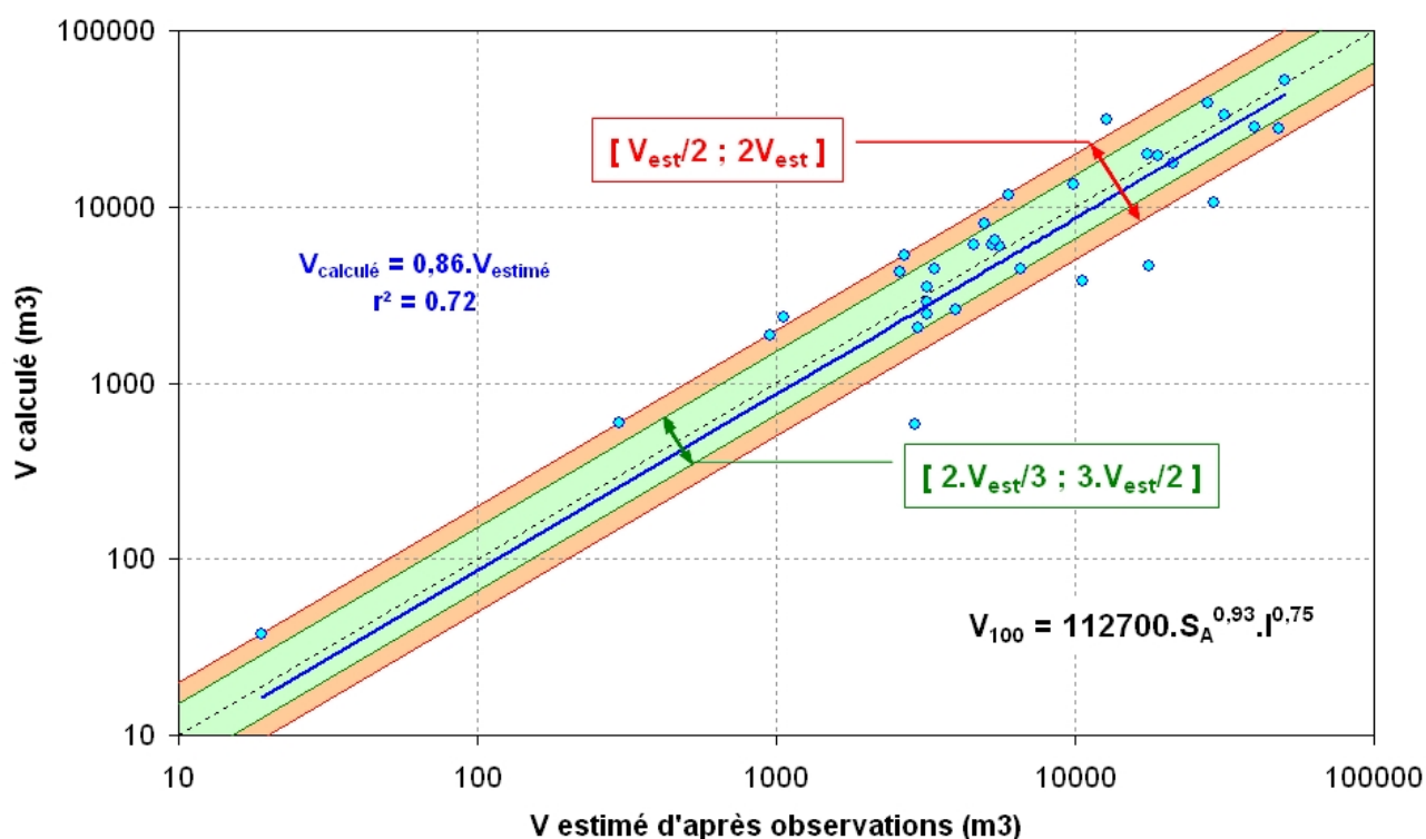
Figure 10. Reconstitution de la production sédimentaire de temps de retour centennal à partir de la relation (2)
