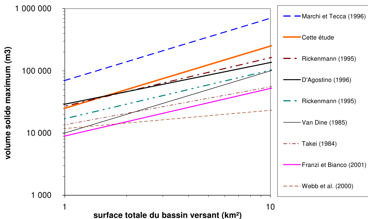
Figure 16. Comparaison de la relation V_{\max} = 25000.S proposée dans cette étude avec des relations similaires publiées par d'autres auteurs
