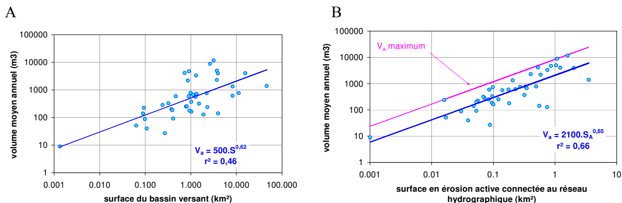
Figure 8. (A) Production sédimentaire en moyenne annuelle en fonction de (A) la taille du bassin versant et (B) de l'étendue des zones en érosion active connectées au réseau hydrographique
