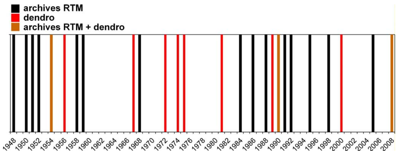
Figure 34. L'enquête dendrogéomorphologique a permis d'inventorier des événements non connus des archives RTM
