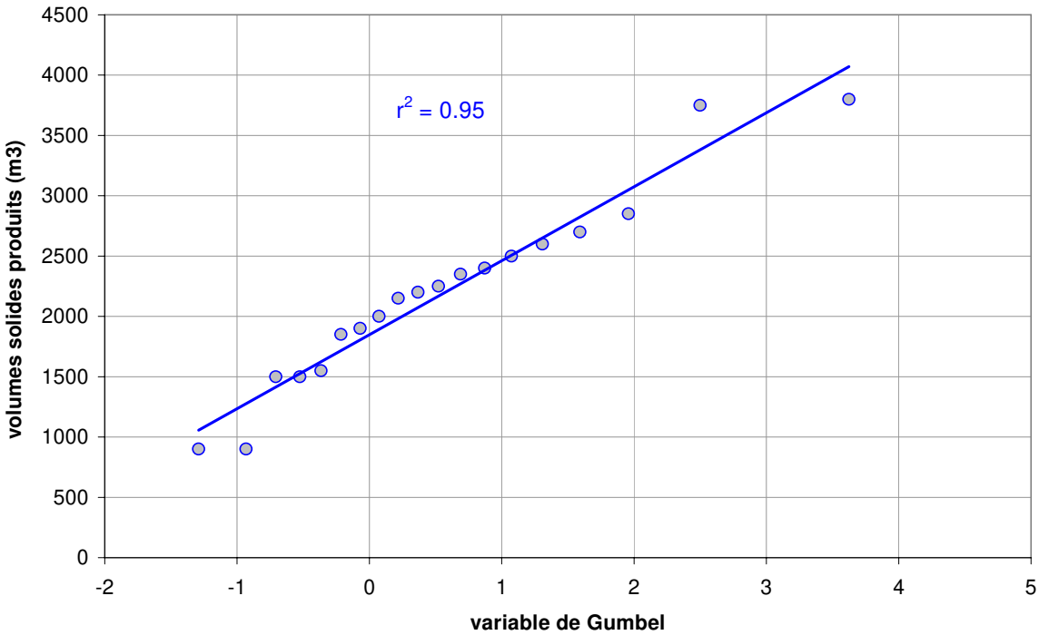
Figure 7. Ajustement statistique des données de production sédimentaire du torrent du Laval (04) à une loi de Gumbel
